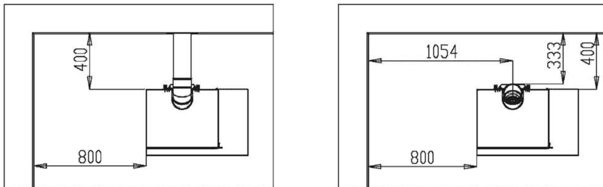
Figure 2 (distances face aux parois en matériau combustible)
