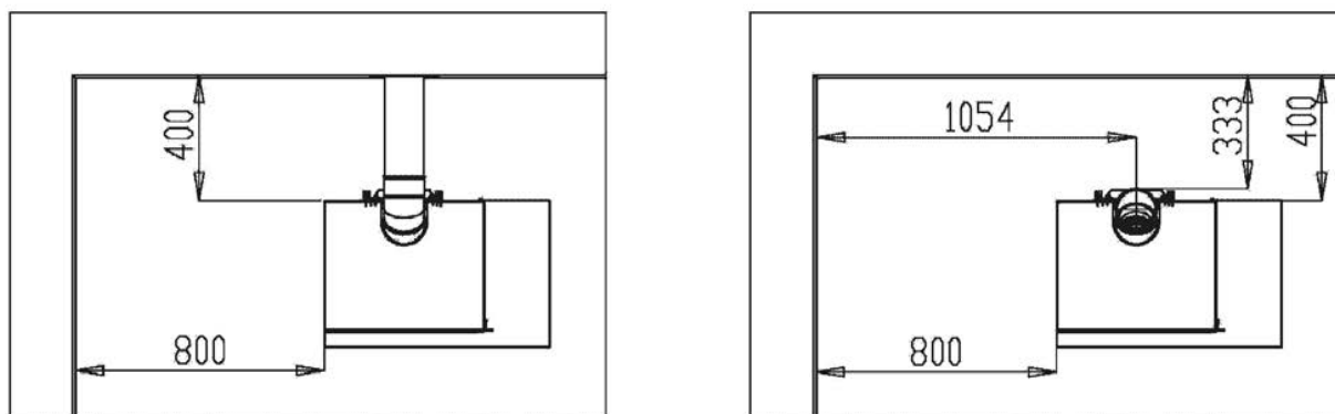
Abbildung 2 (Abstände zu Wänden aus brennbarem Material)
